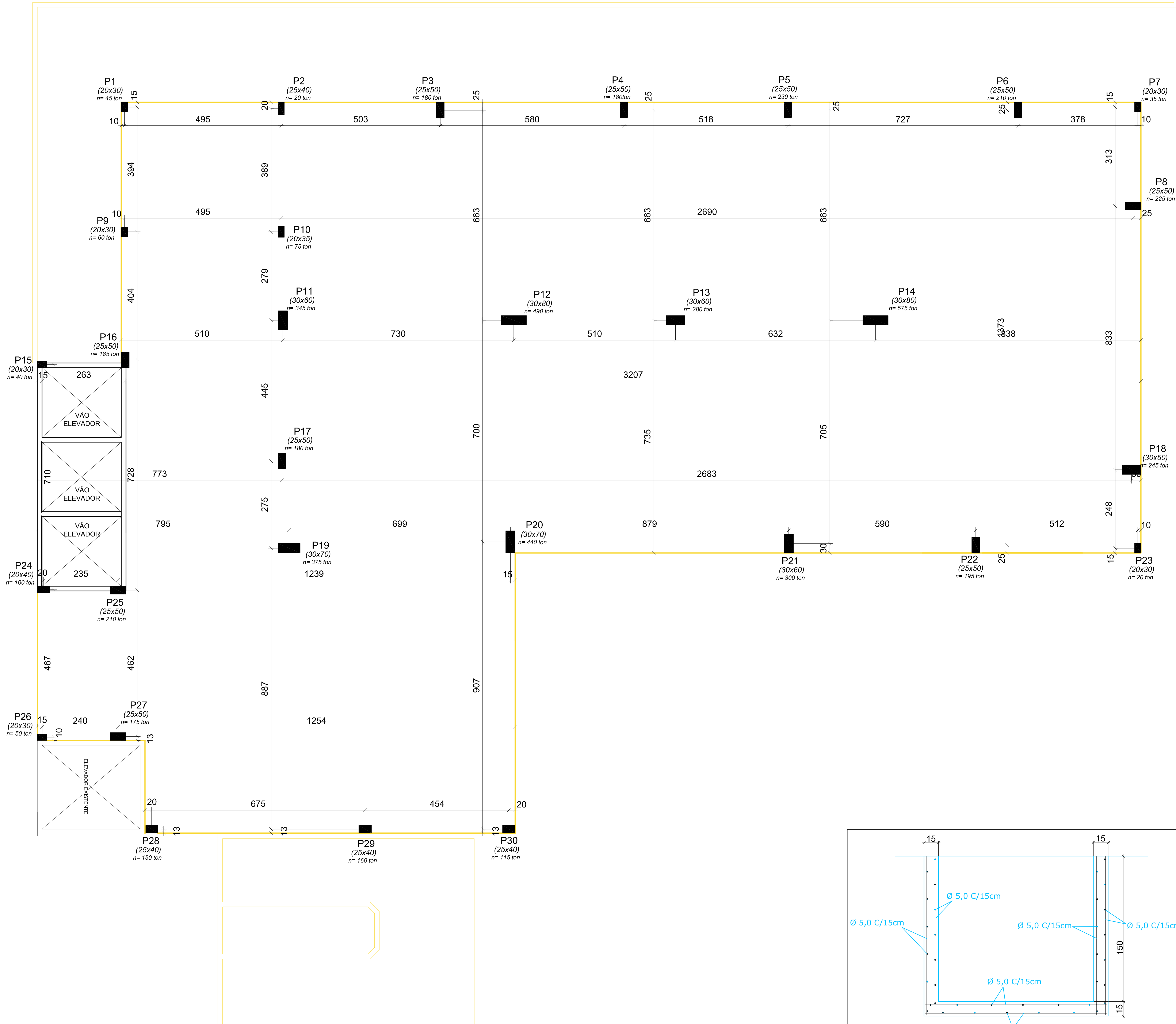
Planta de Locação dos Pilares Escala 1:50
